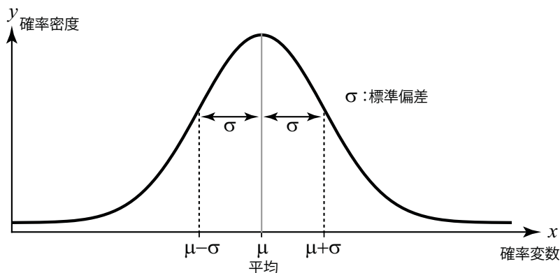
図3: 正規分布
