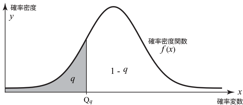
図 6: q 分位数
